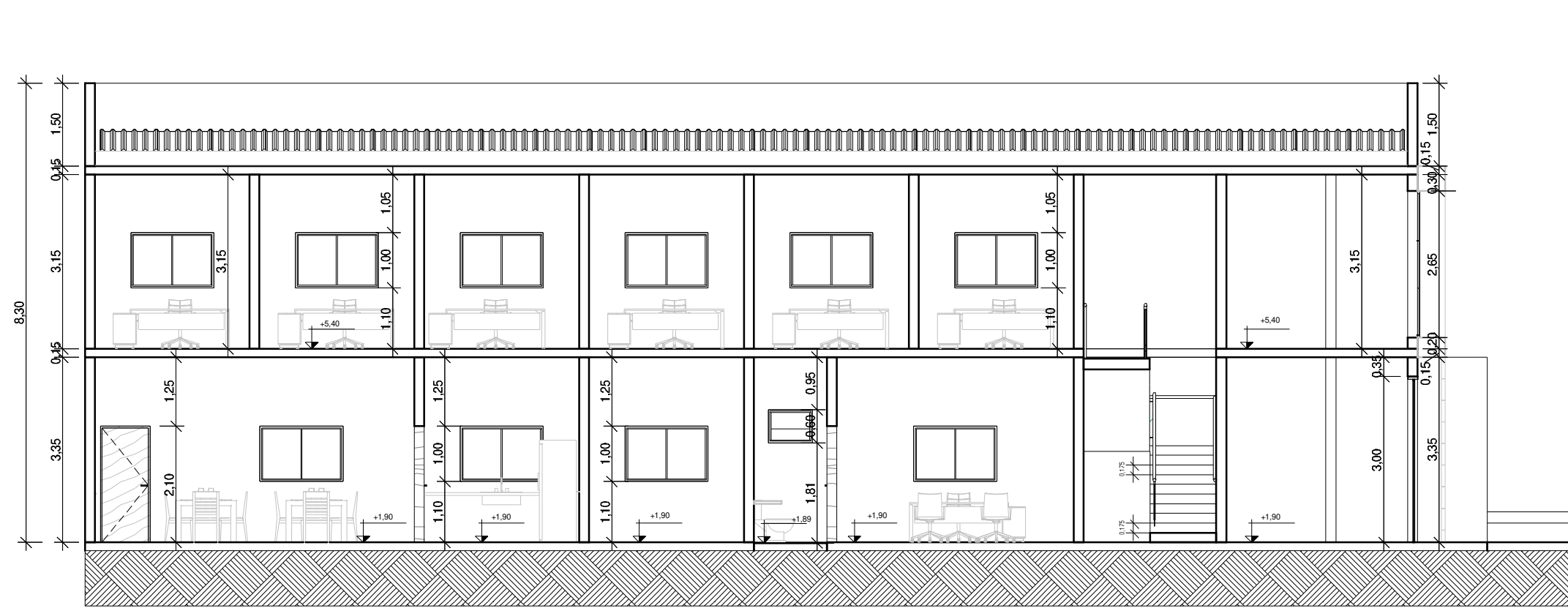
7 CORTE AA Escala: 1 : 100
